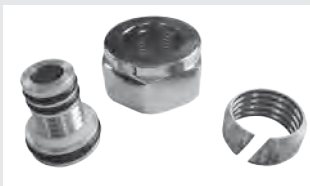
9200133 Aansluitkoppeling M24 - 16 x 2mm, chroom. Voor aluminium-kunststof buis
