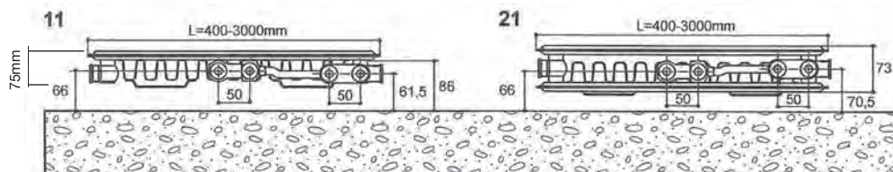
Onderaanzichten Thermrad Super-8 Aangegeven maten uit de muur alleen geldig met bijgeleverde klikconsoles.
