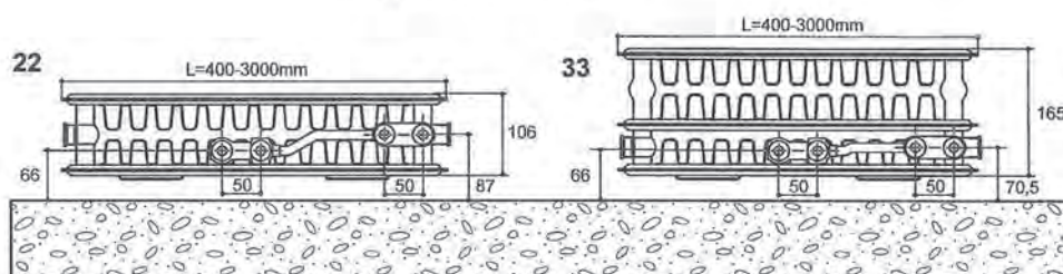
Onderaanzichten Thermrad Super-8 Aangegeven maten uit de muur alleen geldig met bijgeleverde klikconsoles.
